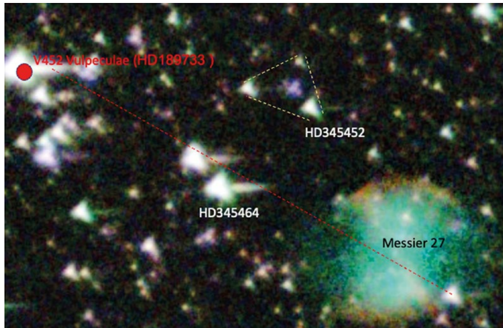
5 Vergrößerter Ausschnitt um M 27 aus Abb. 4. Die Abbildungs- und Auslesefehler werden überdeutlich. Oben links der Veränderliche V452 Vulpeculae (roter Punkt), um den ein Exoplanet kreist (siehe auch Text).
