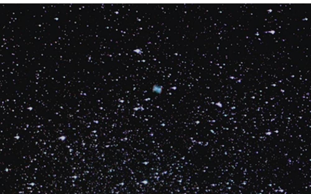
4 Originalbild des Hantelnebels Messier 27 im Sternbild Vulpecula, aufgenommen am 05.11.2024 in Innsbruck, 999 x 15 s belichtet bei Gain 80.
